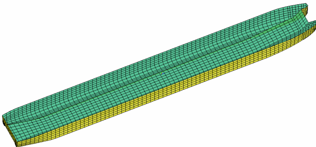
Abb. 57 Diskretisierte Rumpfoberfläche des Semikatamaran-See für die numerischen Seegangsrechnungen
