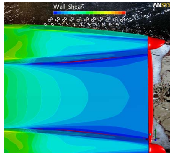
Abb. 25 Wandschubspannungen (Isoflächen)
