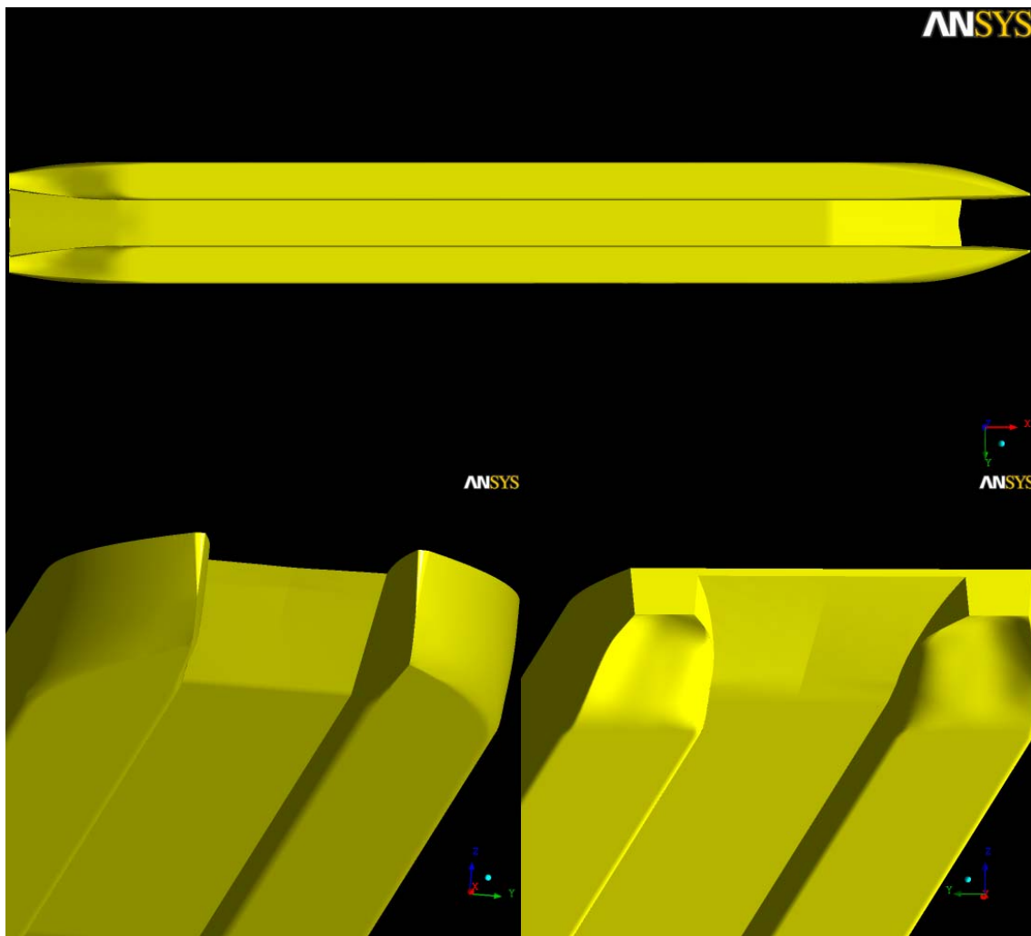
Abb. 30 Geometrie M1793B
