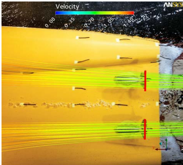
Abb. 26 Stromlinien zum Propeller (Blick von unten)
