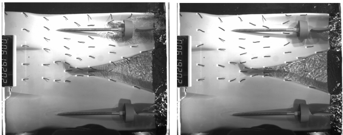
Abb. 56 Pfahlzugversuch bei einer Wassertiefe von 2,1 m und einem Tiefgang von 1,84 m. Bei kleiner Drehzahl läuft der Propeller teilweise in Luft, der Tunnel ist nicht vollständig geflutet (links). Erst bei größerer Drehzahl wird der Tunnel durch die Sogwirkung des Propellers geflutet (rechts). An der Kimm neben der Düse sind Wirbel zu erkennen.
