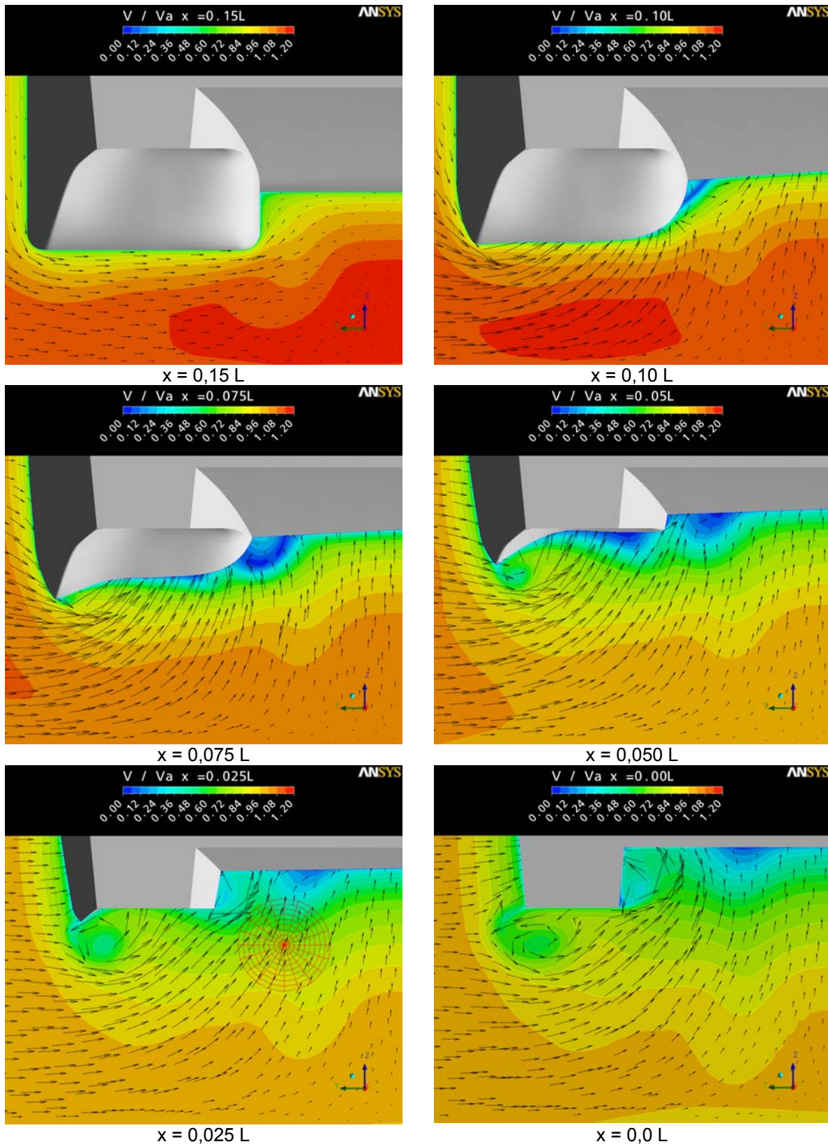
Abb. 35 v/v_{\text{Schiff}} an verschiedenen x-Koordinaten
