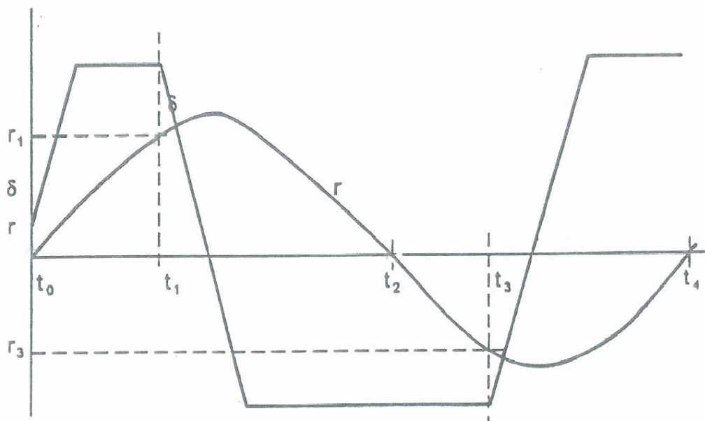
Abb. 75 Schematischer Verlauf eines R-Manövers
