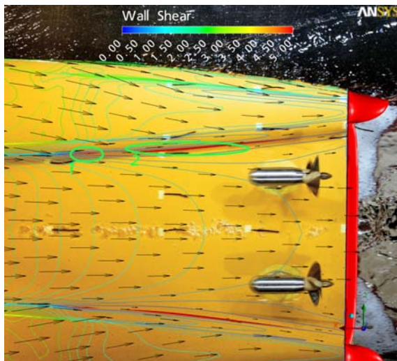
Abb. 24 Wandschubspannungen, (Isolinien)
