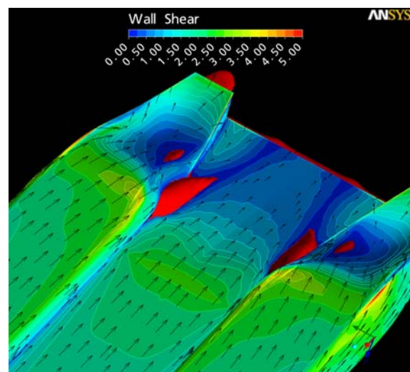
Abb. 32 Mögliche Ablösegebiete M1793B
