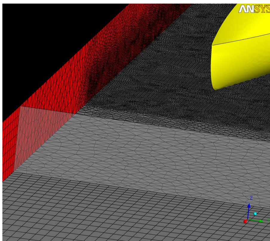
Abb. 20 Kopplung Hybridgitter
