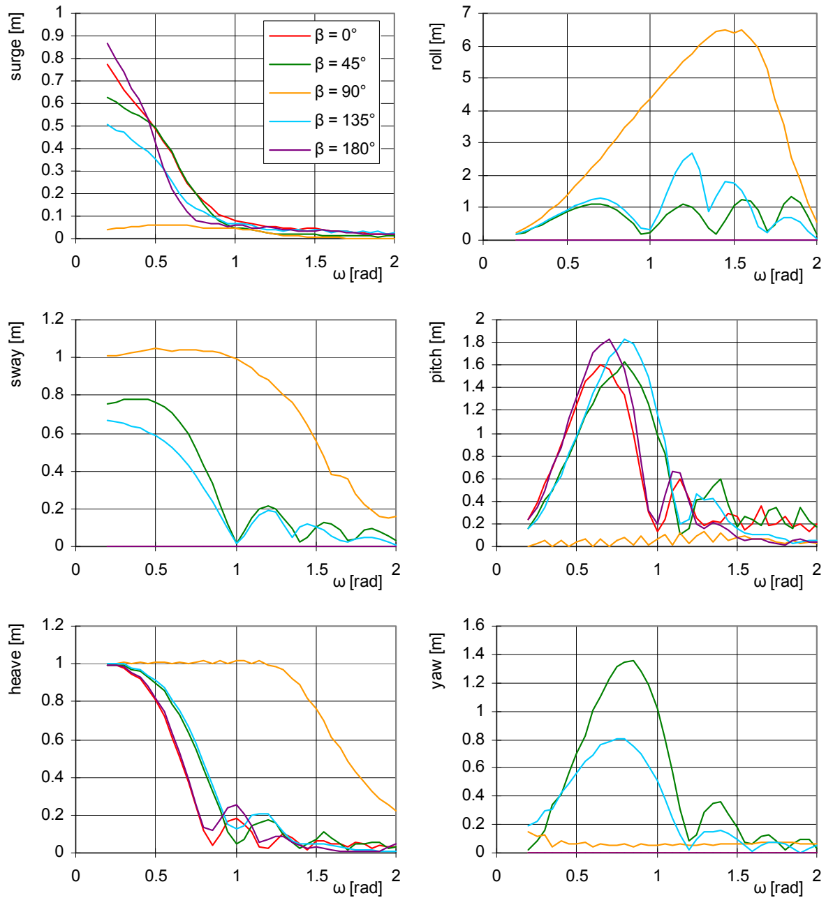
Abb. 98 Übertragungsfunktionen für ein vergleichbares Küstenmotorschiff bei einer Verdrängung von 1565 m 3 und einer Geschwindigkeit von 2,8 m/s.
