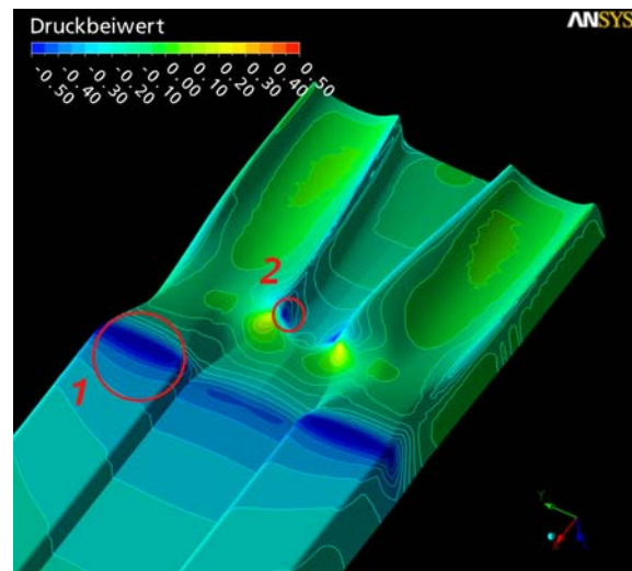
Abb. 46 Mögliche Ablösegebiete M1793E
