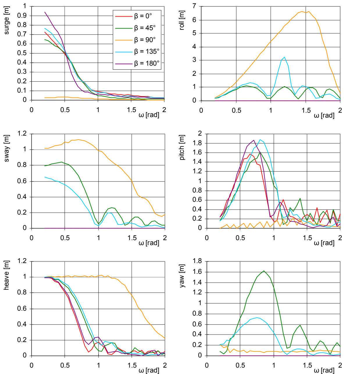
Abb. 96 Übertragungsfunktionen für ein vergleichbares Küstenmotorschiff bei einer Verdrängung von 1565 m 3 und einer Geschwindigkeit von 4,2 m/s.
