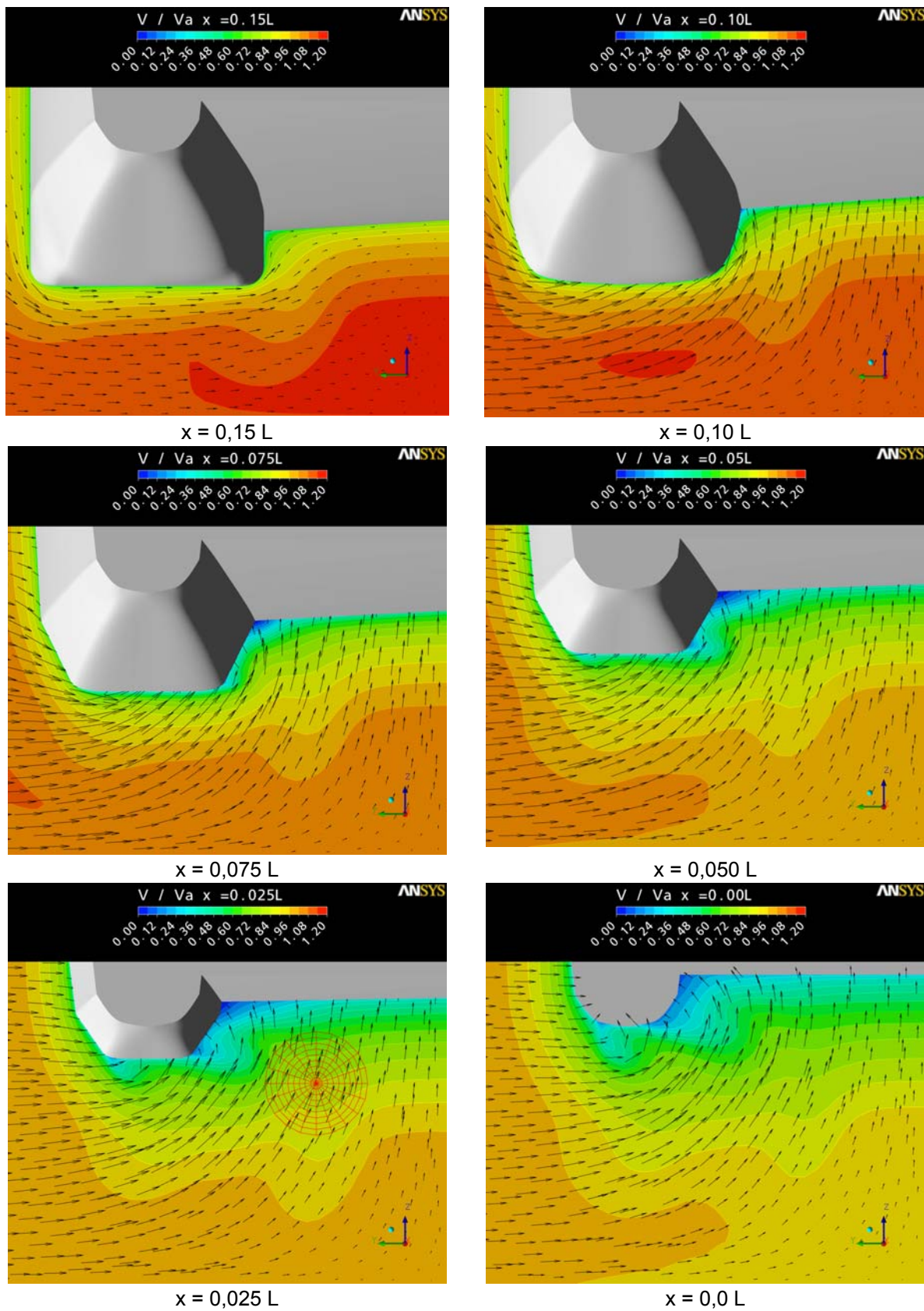
Abb. 28 v/v_{\text{Schiff}} an verschiedenen x-Koordinaten
