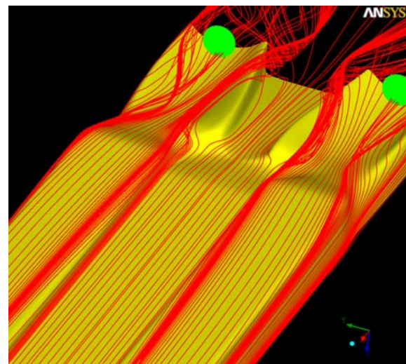
Abb. 48 Stromlinien am Schiffsrumpf
