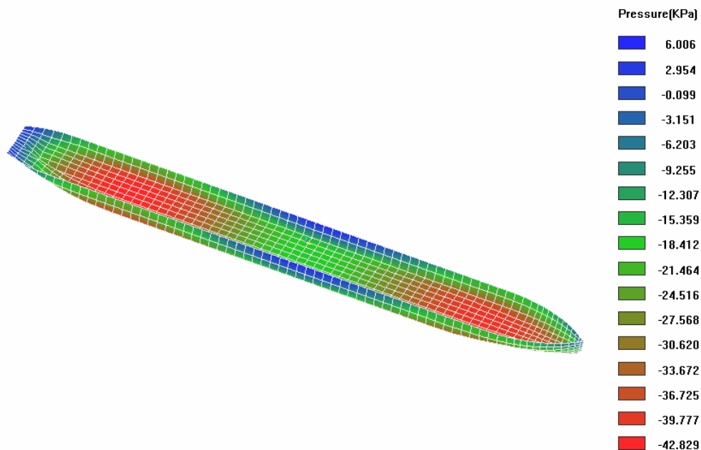
Abb. 62 Beispielhafte Druckverteilung auf dem Küstenmotorschiff, (Verdrängung 3282 m 3 , Geschwindigkeit = 5,6m/s, Welleneinfallswinkel = 135°, Wellenfrequenz = 1,0 s -1 , Wellenphase = 180°)
