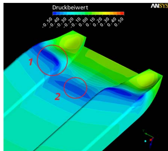
Abb. 38 Druckbeiwerte M1793B
