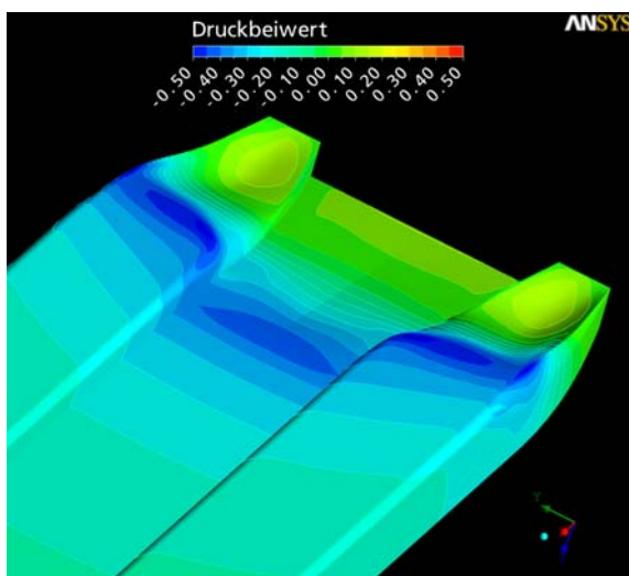
Abb. 31 Druckbeiwerte M1793B
