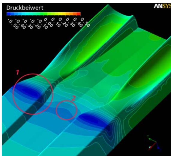
Abb. 37 Druckbeiwerte M1793C
