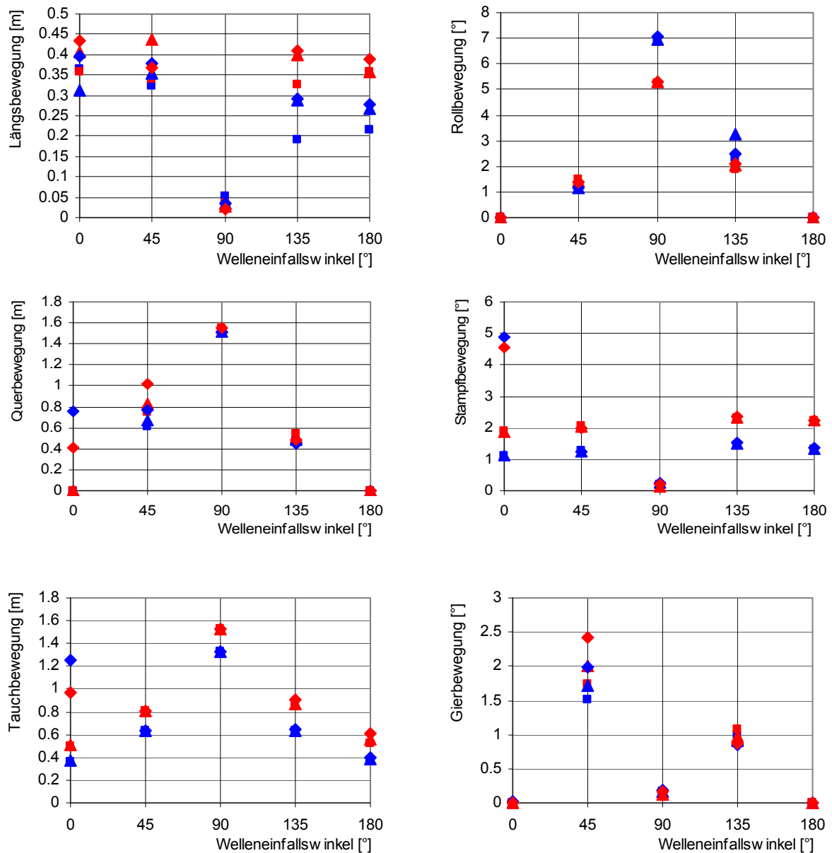
Abb. 64 Berechnete signifikante Bewegungen für den Semikatamaran-See und eine vergleichbares Küstenmotorschiff bei einer Verdrängung von 1565 m³ und einer Windgeschwindigkeit von 12 m/s. Die Ergebnisse für den Semikatamaran-See sind blau dargestellt, die für ein vergleichbares Küstenmotorschiff rot; Geschwindigkeiten: □ = 2,8 m/s, △ = 4,2 m/s und ◇ = 5,6 m/s.
