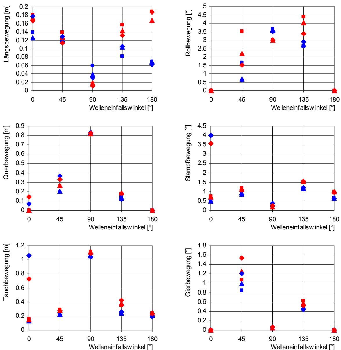
Abb. 65 Berechnete signifikante Bewegungen für den Semikatamaran-See und eine vergleichbares Küstenmotorschiff bei einer Verdrängung von 3282 m 3 und einer Windgeschwindigkeit von 10 m/s. Die Ergebnisse für den Semikatamaran-See sind blau dargestellt, die für ein vergleichbares Küstenmotorschiff rot; Geschwindigkeiten: □ = 2,8 m/s, △ = 4,2 m/s und ◇ = 5,6 m/s.
