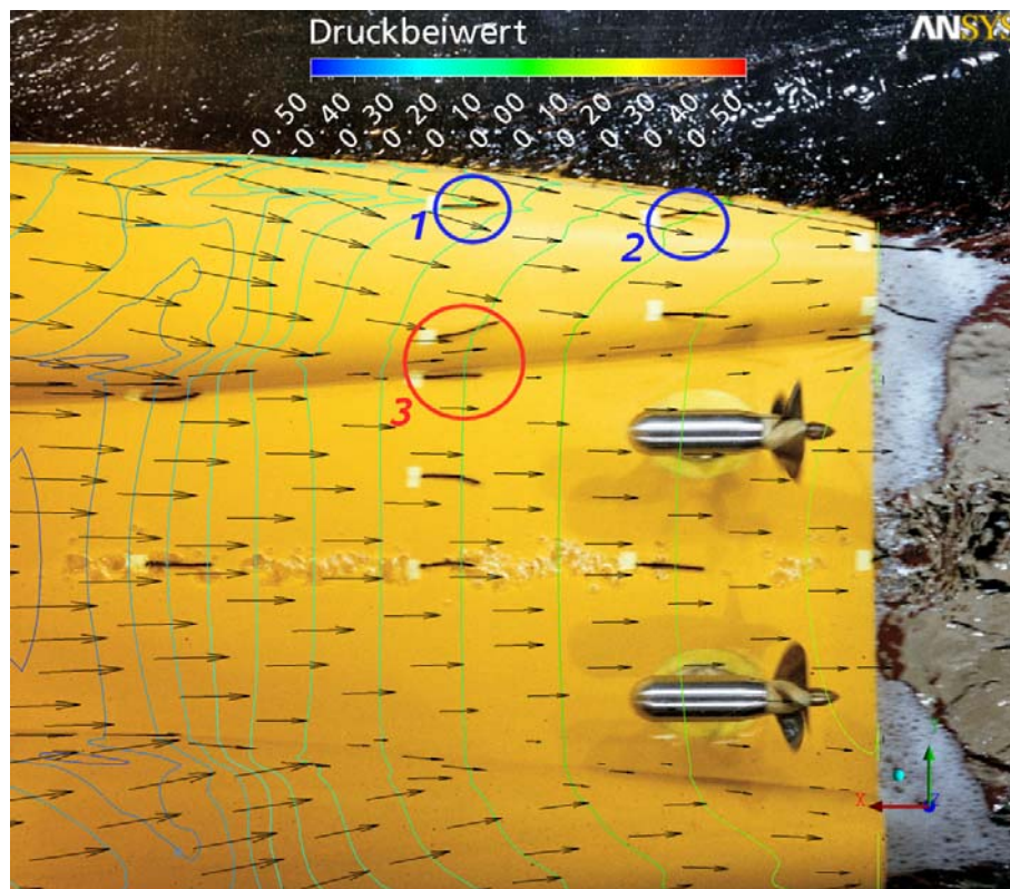
Abb. 23 Vergleich Stromfadenversuch mit numerischen Ergebnissen für M1772
