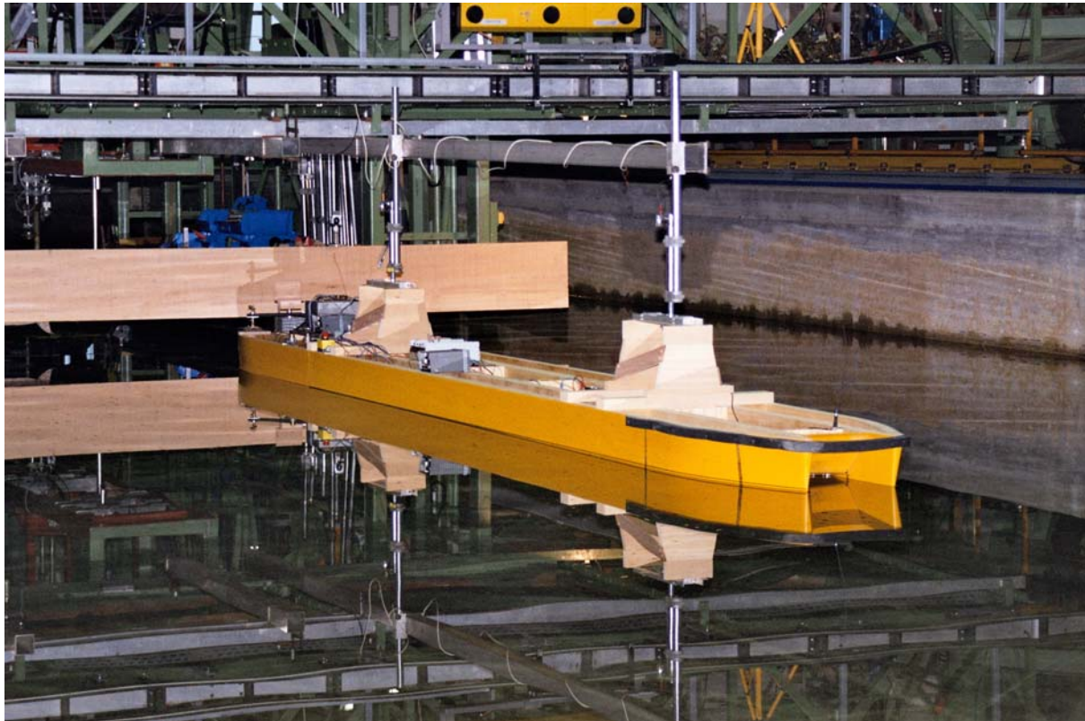
Abb. 74 Modell M1772 vor dem Beginn der Messfahrt; während der Fahrt fährt das Modell frei.
