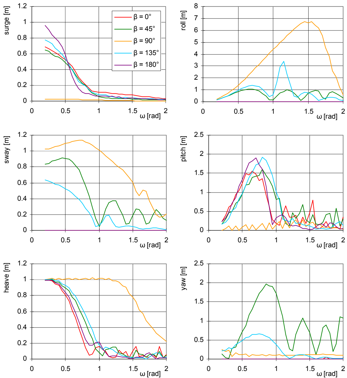
Abb. 94 Übertragungsfunktionen für ein vergleichbares Küstenmotorschiff bei einer Verdrängung von 1565 m 3 und einer Geschwindigkeit von 5,6 m/s.
